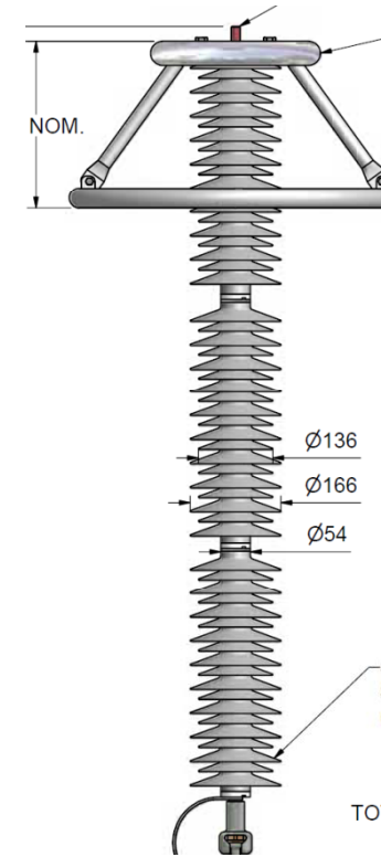
Pararrayos para líneas de Transmisión
